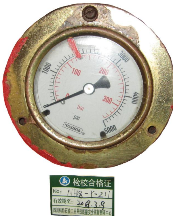
Рисунок 1 – Внешний вид манометра деформационного показывающего 25-310-5000
