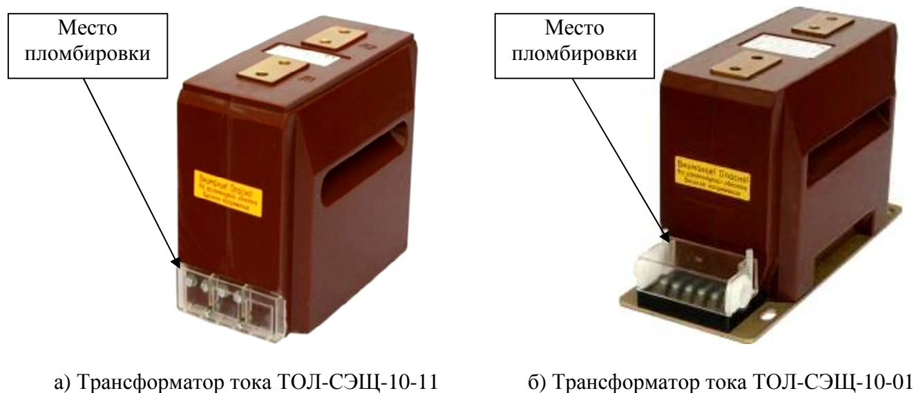
Рисунок 1 - Общий вид средства измерений и схема пломбировки от несанкционированного доступа
