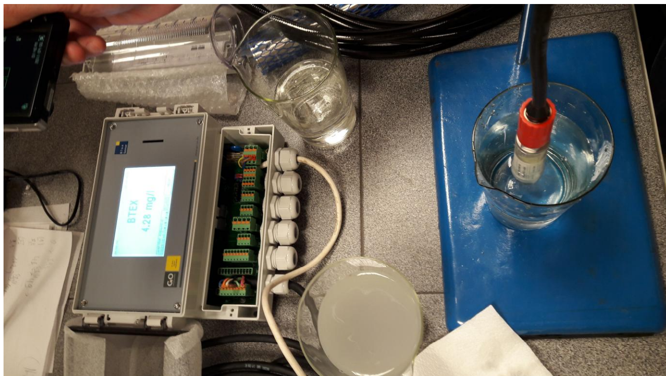
Рисунок 1 - Общий вид анализатора в конфигурации (вычислительный модуль BlueSense - погружной датчик нефтепродуктов)
