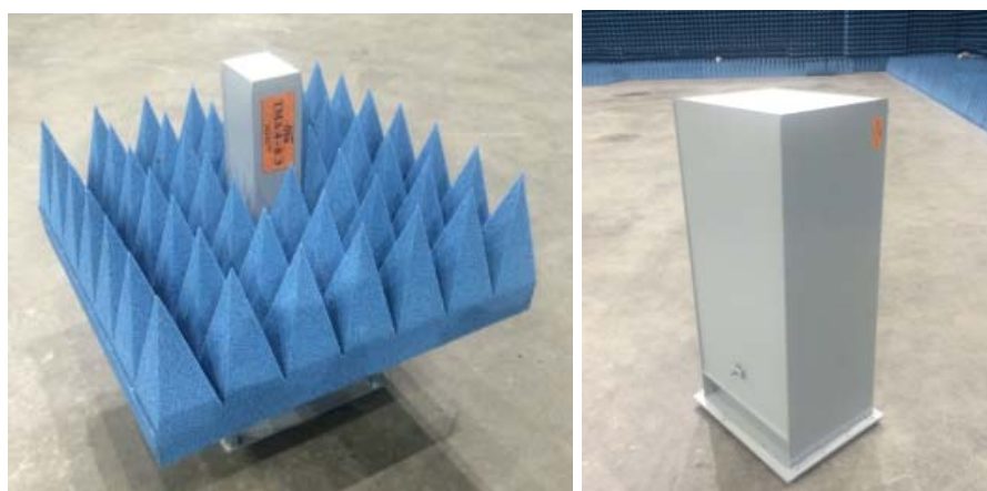
Рисунок 6 - Внешний вид антенны-зонда ТМАЗ 4-6 И диапазона частот 4 - 6 ГГц (слева), внешний вид антенны ТМА 1-6 Э (справа)
