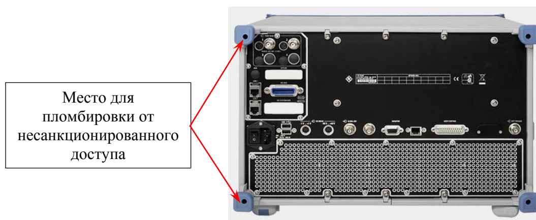
Рисунок 8 - Задняя панель векторного анализатора цепей ZVA 8
