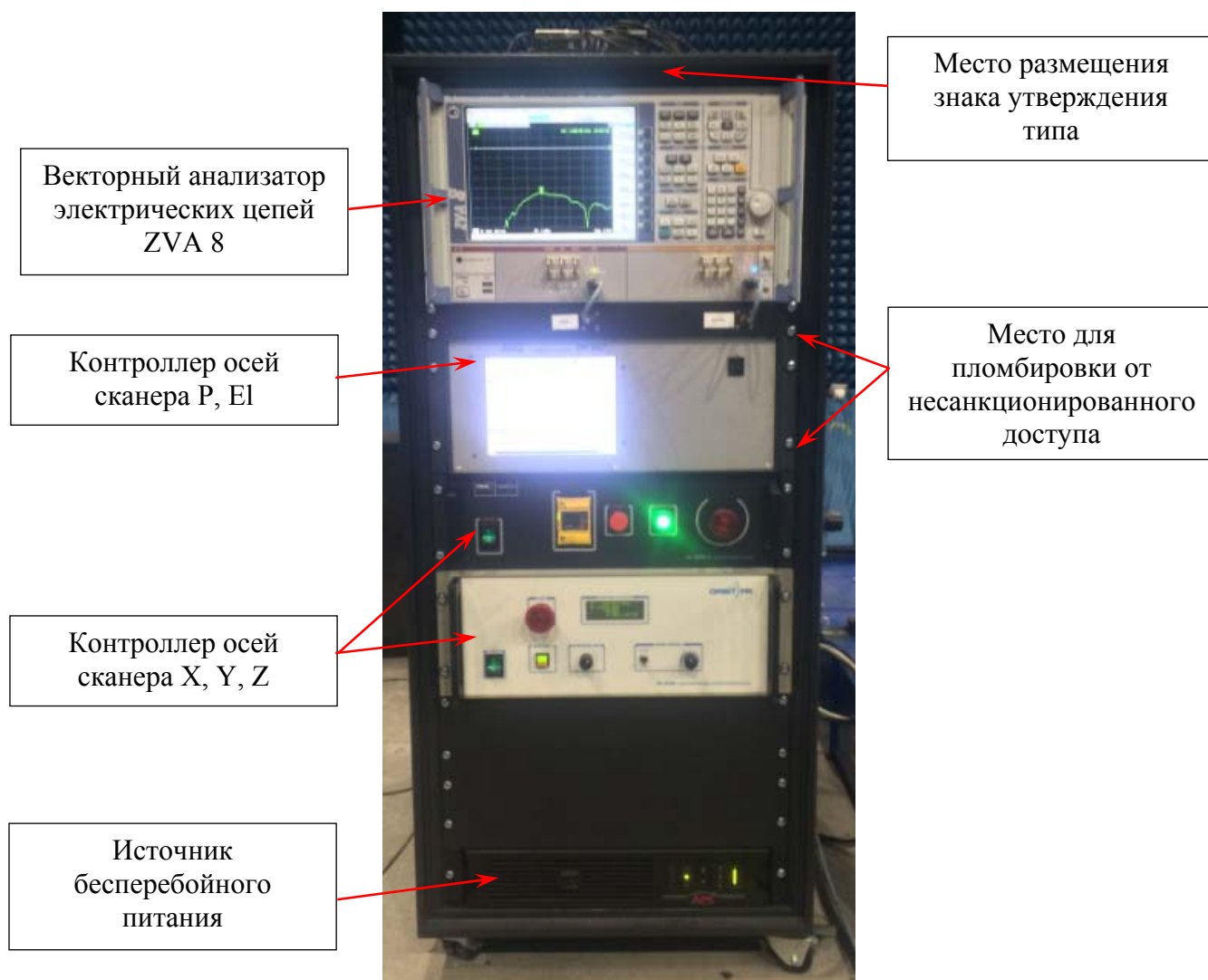
Рисунок 7 - Внешний вид приборной стойки для размещения элементов комплекса и места размещения знака утверждения типа
