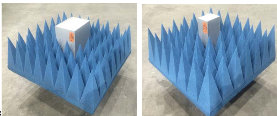
Рисунок 5 - Внешний вид антенны-зонда ТМАЗ 1-2 И диапазона частот 1 - 2 ГГц (слева), внешний вид антенны-зонда ТМАЗ 2-4 И диапазона частот 2 - 4 ГГц (справа)
