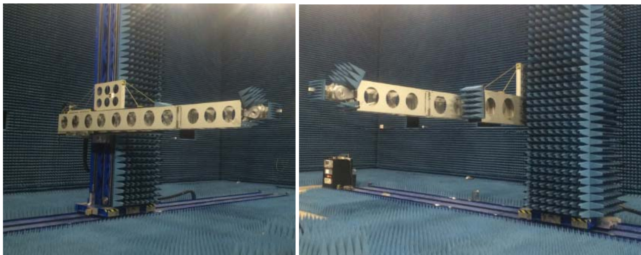
Рисунок 1 - Общий вид конструкции сканера AL-4953-1-13m-13m-V-S
