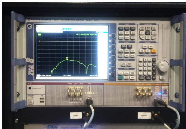
Рисунок 4 - Внешний вид векторного анализатора электрических цепей ZVA
