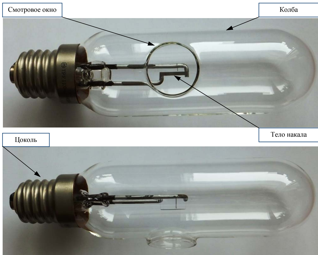
Рисунок 1 - Общий вид излучателей на основе ламп ТРУ
