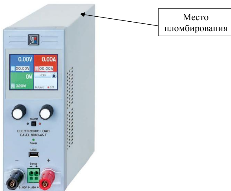
Рисунок 4 - Общий вид и место пломбирования нагрузок серии EA-EL 9000 T
