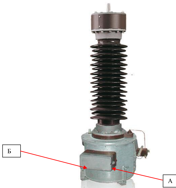
Рисунок 1 - Общий вид трансформатора напряжения емкостного DDB-123
