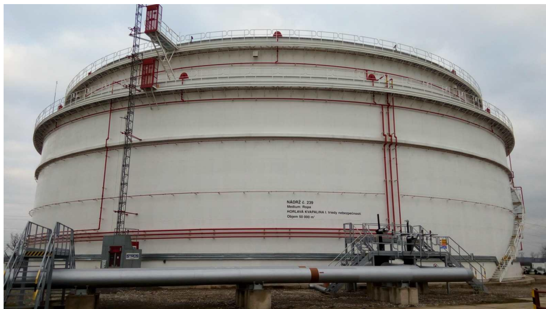
Рисунок 2 - Общий вид резервуара РВСПК-50000
