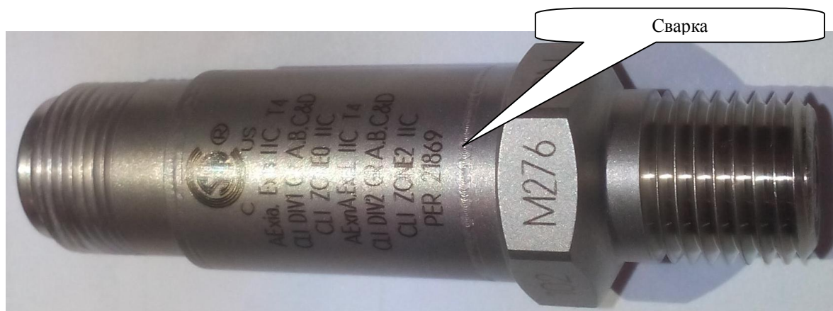
Рисунок 1 - Внешний вид датчика динамического давления ICP модели 102M276
