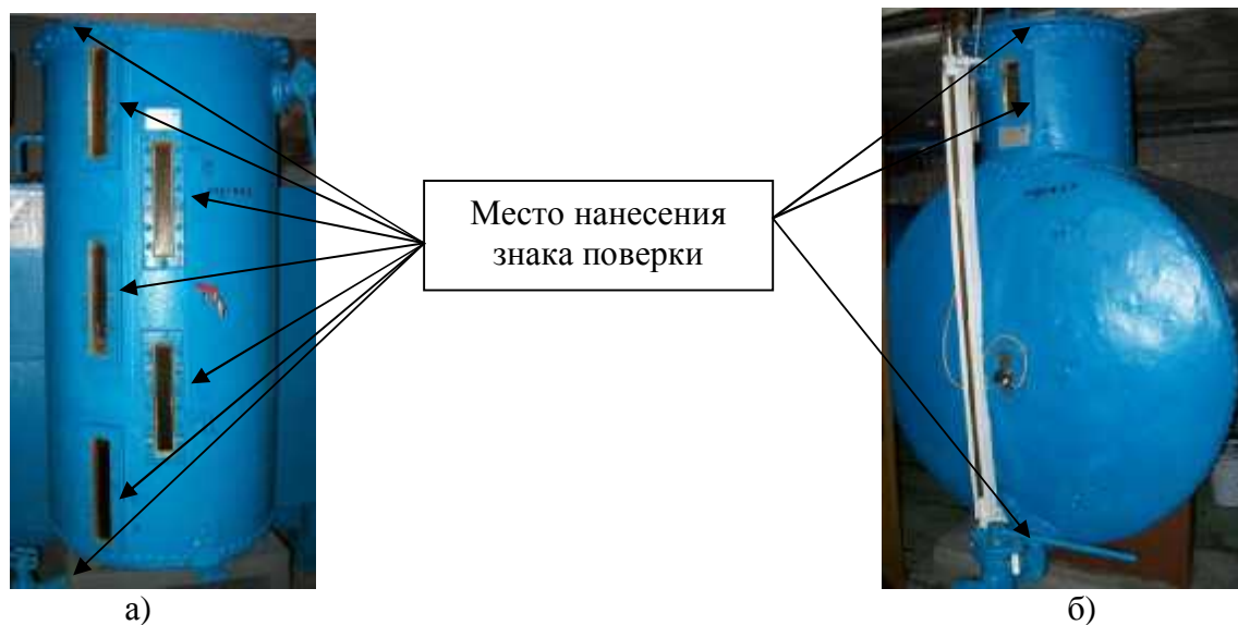
Рисунок 3 - Схема пломбировки от несанкционированного доступа, обозначение места нанесения знака поверки мерников а) ММВ, б) ММГ
