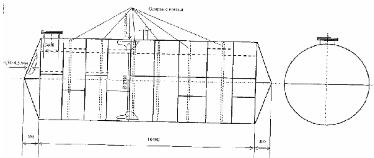
Рисунок 2 - Эскиз резервуара горизонтального стального цилиндрического РГС-65
