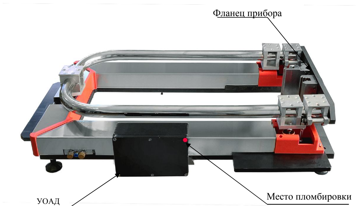
Рисунок 1 -Общий вид измерительного блока
