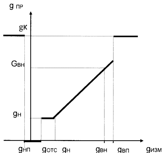
Рисунок 4.3 – Преобразование измеренных значений массового расхода
