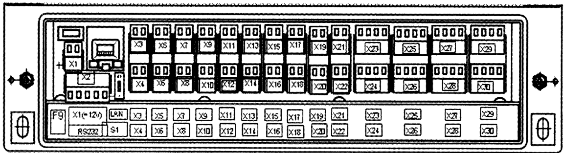
Рисунок 3.2 - Монтажный отсек (крышка снята)
