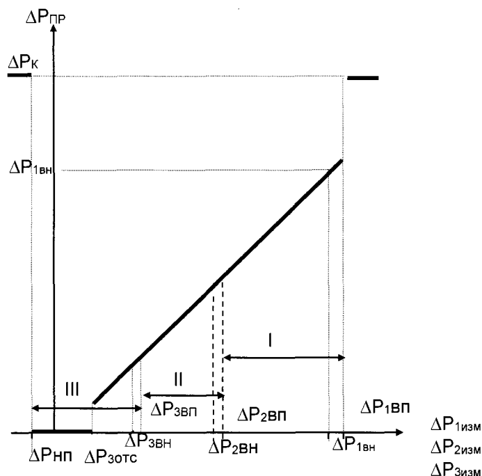
Рисунок 4.6 – Преобразование значений перепада давления, измеренных тремя датчиками
