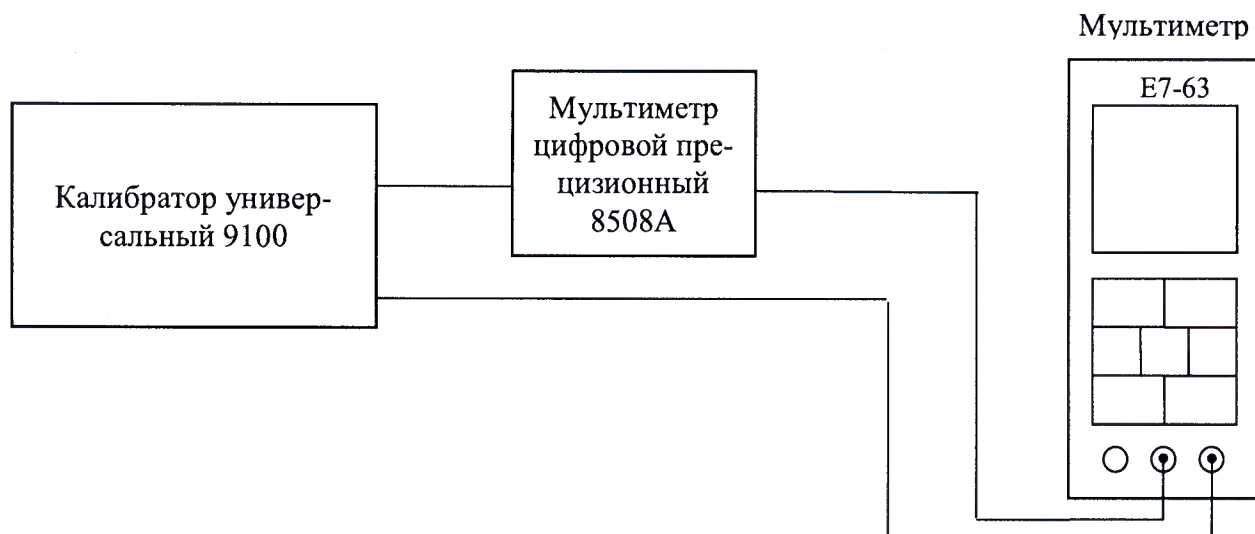
Рисунок 2 – Структурная схема опробования и определения приведенной (к верхнему значению диапазона измерений) погрешности измерений силы* переменного тока
