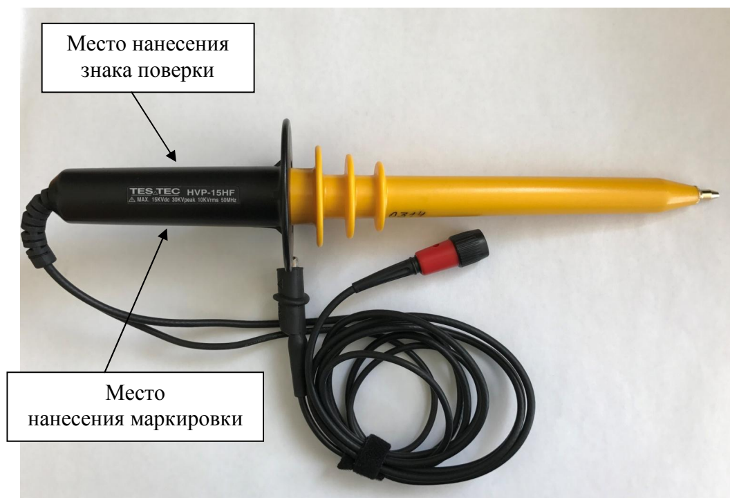
Рисунок 2 - Обозначение места нанесения маркировки, знака поверки
