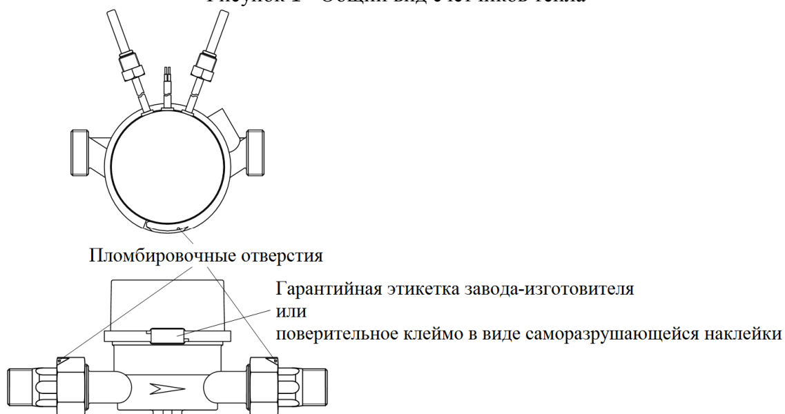
Рисунок 1 - Общий вид счетчиков тепла
