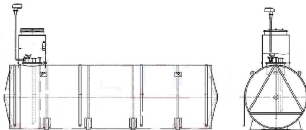
Рисунок 1 - Общий вид эскиза резервуаров РГС-10, РГС-40
