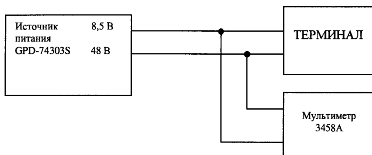
Рисунок 3 – Схема подключения приборов для определения абсолютной погрешности измерений напряжения постоянного тока внешнего питания
