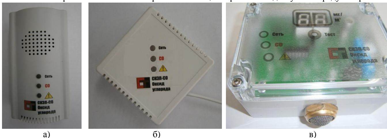
Рисунок 1 – Фотография общего вида сигнализаторов загазованности а) СКЗП-СО-1, б) СКЗП-СО-2, в) СКЗП-СО-3.
