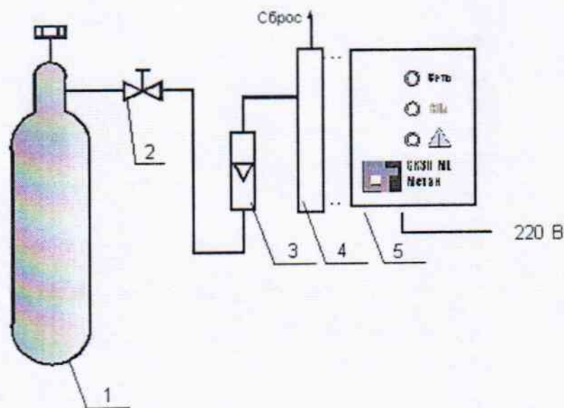
1 – баллон с ГСО-ПГС; 2 – вентиль точной регулировки; 3 – индикатор расхода; 4 – насадка (показана условно); 5 – сигнализатор
