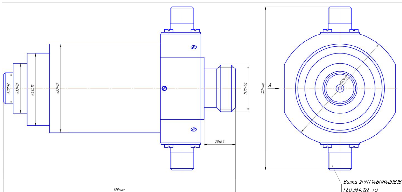
Рисунок 2 – Габаритно-установочные размеры датчика НТ 049
