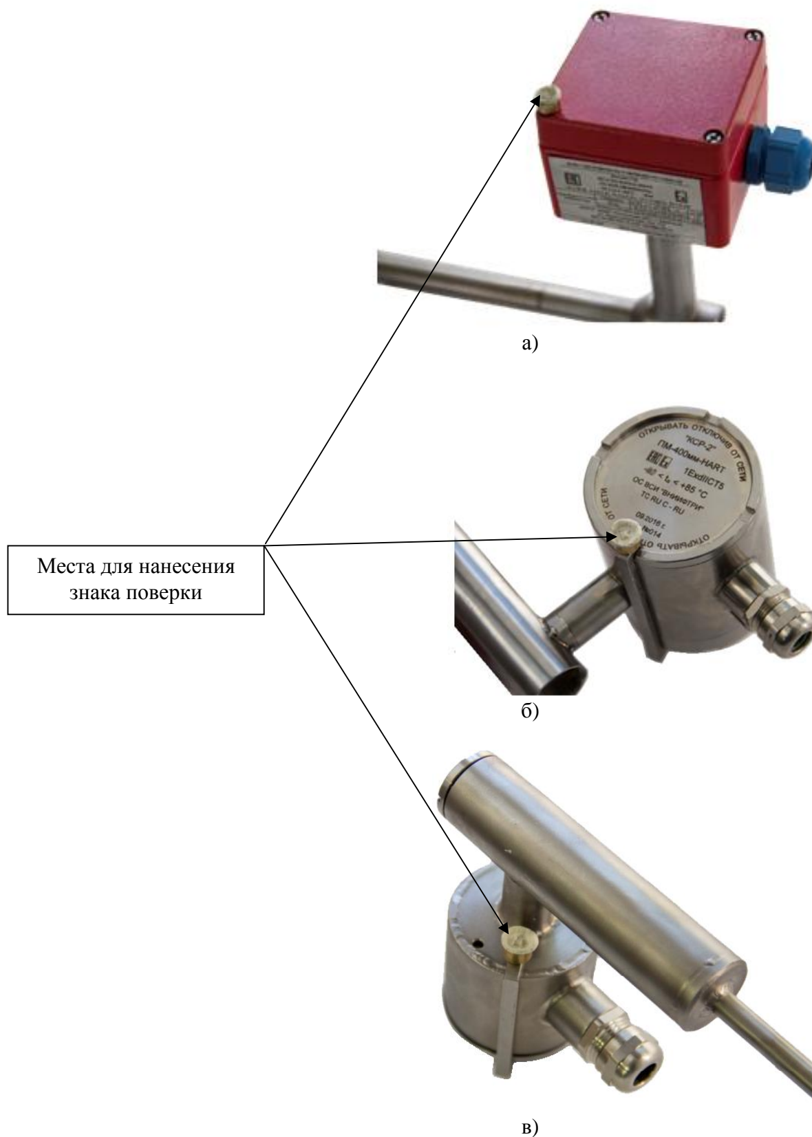
Рисунок 2 - Схема пломбировки от несанкционированного доступа, обозначение мест нанесения знака поверки
