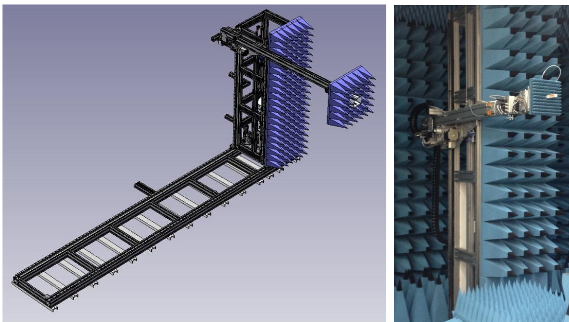
Рисунок 1 – Конструкция и внешний вид сканера с установленной антенной-зондом
