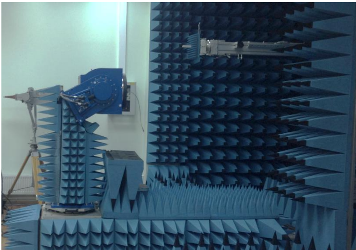
Рисунок 3 – Внешний вид ОПУ и сканера с установленной антенной-зондом
