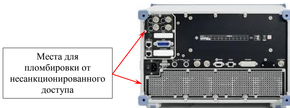
Рисунок 13 – Задняя панель векторного анализатора цепей
