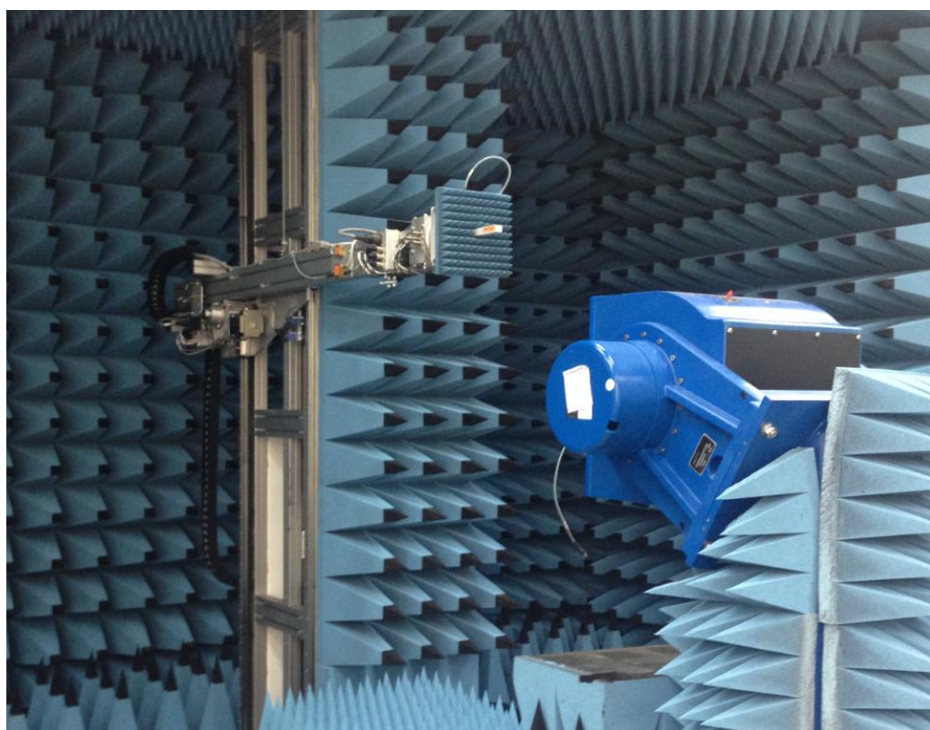
Рисунок 2 – Внешний вид сканера и ОПУ
