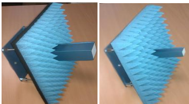
Рисунок 7 – Внешний вид антенн-зондов диапазона частот от 4 до 18 ГГц
