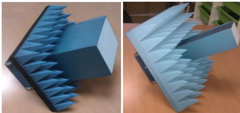
Рисунок 6 – Внешний вид антенн-зондов диапазона частот от 1 до 4 ГГц
