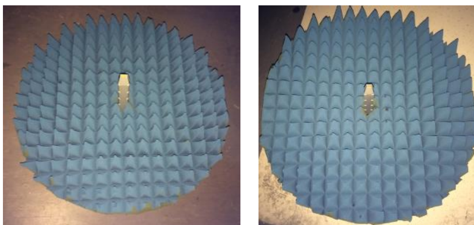
Рисунок 7 - Внешний вид антенн-зондов 42EW и 28EW соответственно
