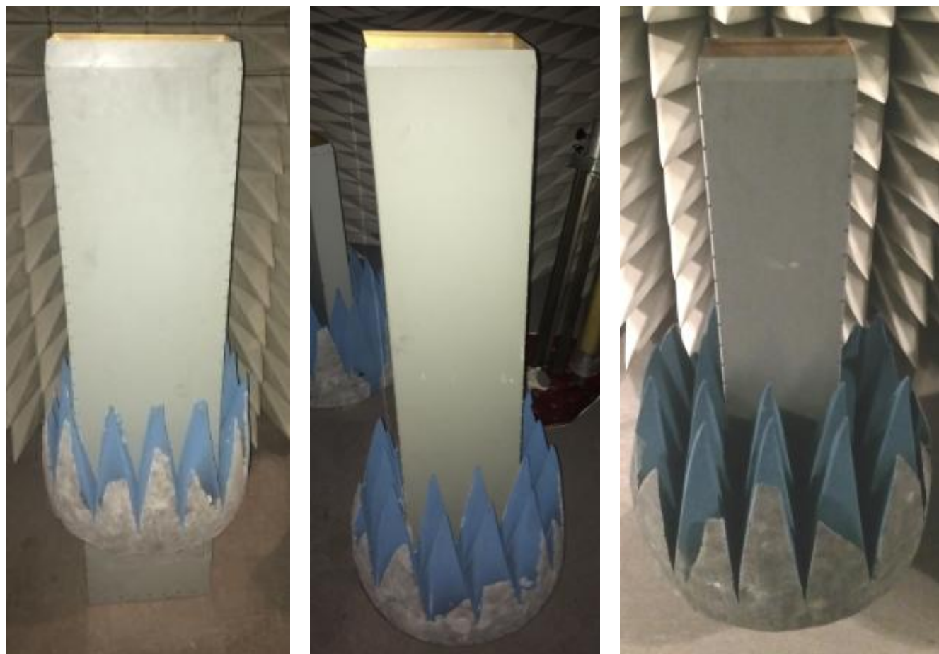
Рисунок 4 - Внешний вид антенн-зондов 975EW, 770EW и 510EW соответственно
