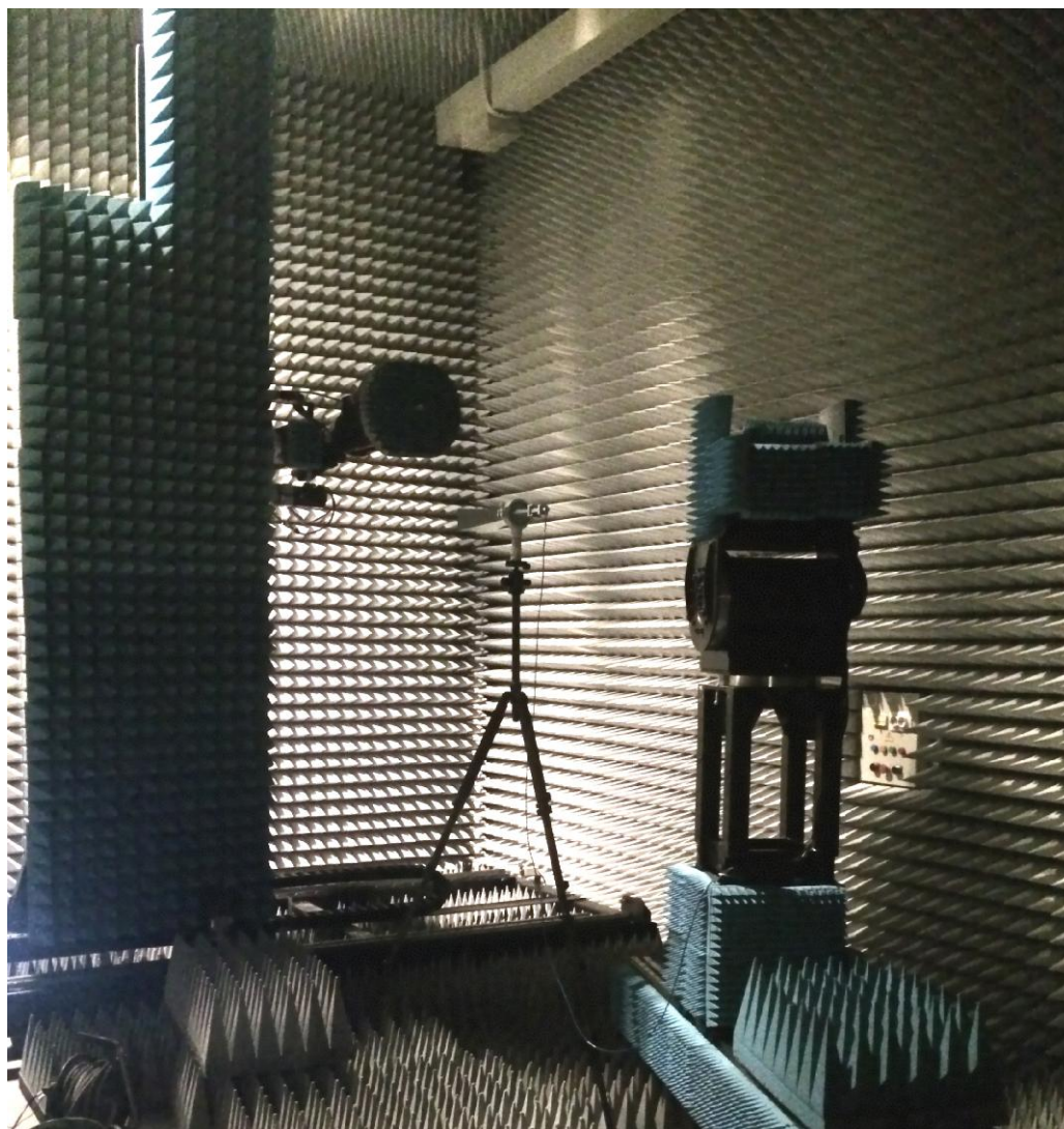
Рисунок 1 - Общий вид комплекса
