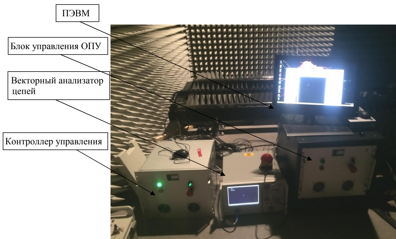
Рисунок 3 - Внешний вид векторного анализатора цепей, контроллера управления, блока управления ОПУ и ПЭВМ
