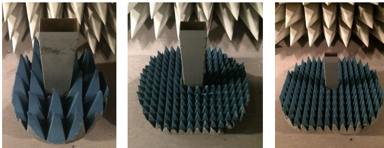
Рисунок 5 - Внешний вид антенн-зондов 340EW, 229EW и 159EW соответственно
