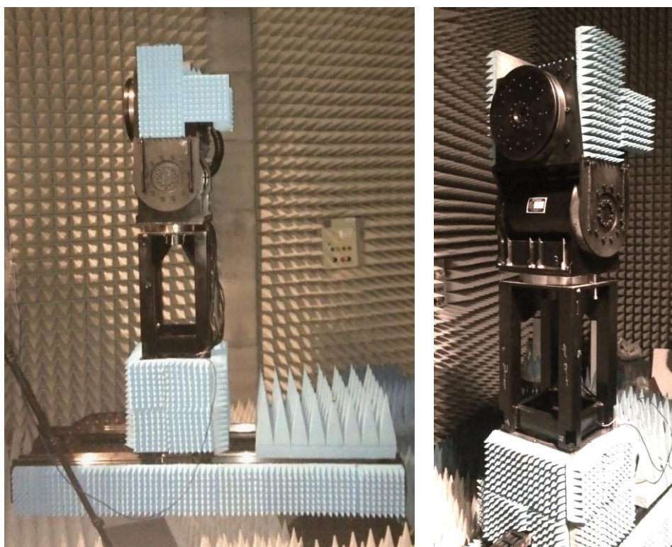
Рисунок 2 - Внешний вид ОПУ
