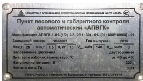
Рисунок 2 - Маркировочная табличка АПВГК
