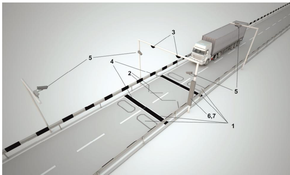
Рисунок 1 - Общий вид АПВГК
