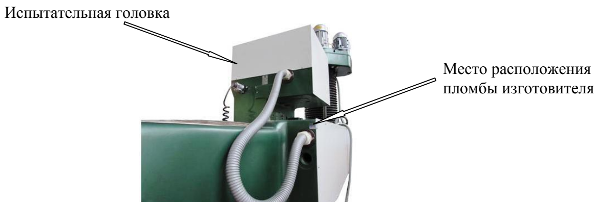
Рисунок 2 - Задняя панель испытательной головки твердомера
