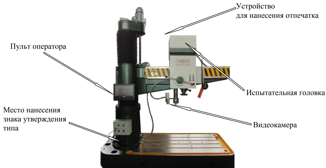
Рисунок 1 - Внешний вид твердомера
