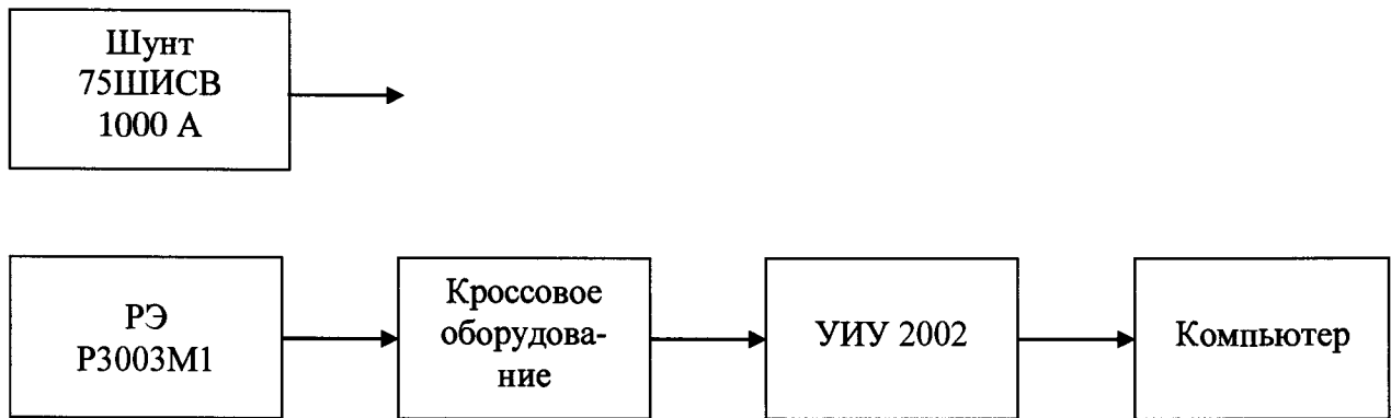
Рисунок 19 - Блок-схема поверки ИК силы постоянного тока запуска ВСУ
