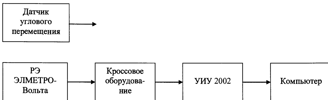
Рисунок 16 - Блок-схема поэлементной поверки ИК угловых перемещений
