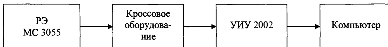
Рисунок 6 - Блок-схема поверки ИК сопротивления постоянному току, соответствующего значениям температуры, в диапазоне от 0 до 200 Ом
