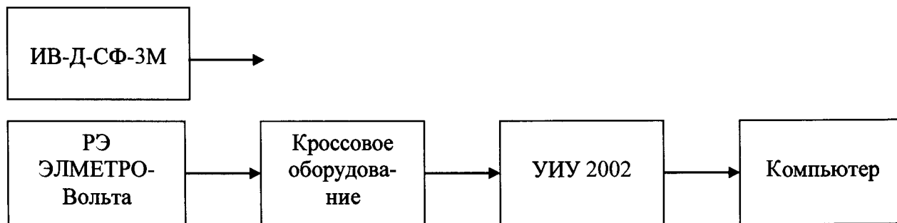
Рисунок 12 - Блок-схема поверки ИК виброскорости и силы постоянного тока, соответствующей значениям виброскорости
