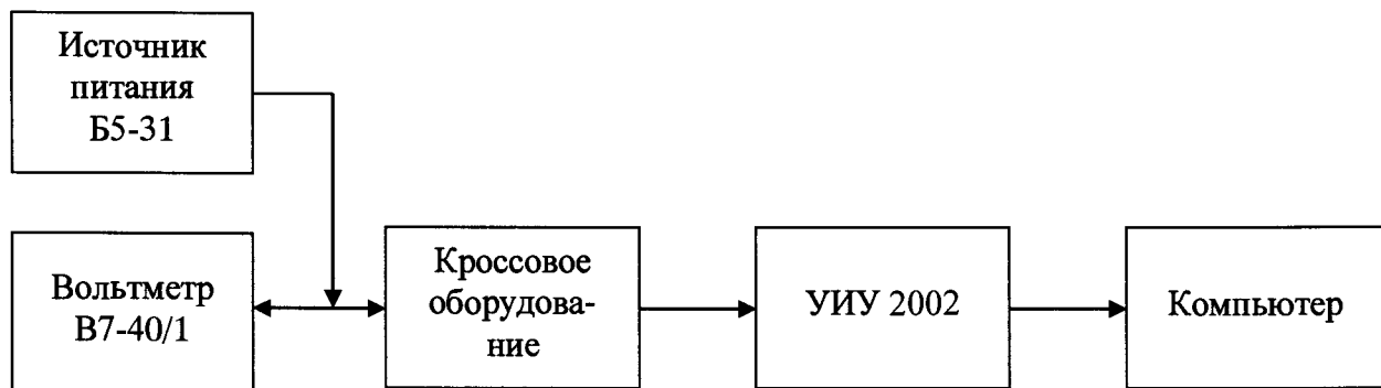
Рисунок 20 - Блок-схема поверки ИК напряжения постоянного тока
