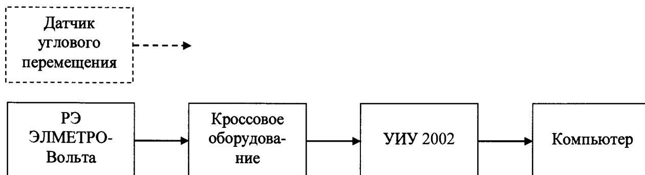
Рисунок 17 - Блок-схема поверки ИК силы постоянного тока, соответствующей значениям углового перемещения
