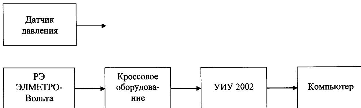
Рисунок 2 - Блок-схема поэлементной поверки ИК давления
