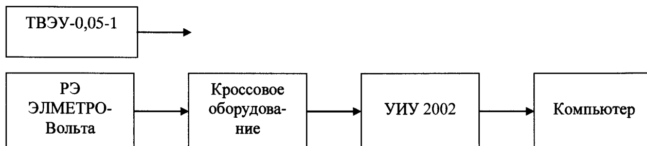
Рисунок 14 - Блок-схема поэлементной поверки ИК массы масла
