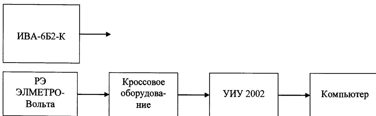
Рисунок 21 - Блок-схема поверки ИК относительной влажности воздуха и ИК температуры датчиков влажности
