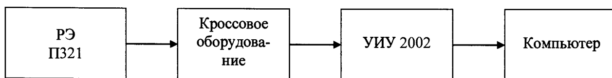
Рисунок 18 - Блок-схема поверки ИК силы постоянного тока, соответствующей значениям углового перемещения, в диапазоне от 4 до 20 мА
