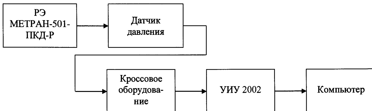
Рисунок 1 - Блок-схема комплектной поверки ИК давления
