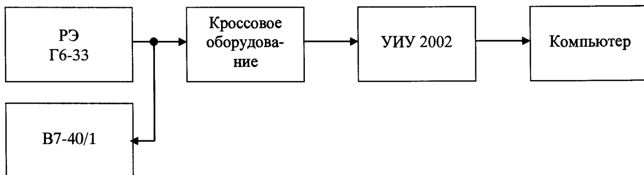
Рисунок 9 - Блок-схема поверки ИК частоты вращения роторов и частоты переменного тока
