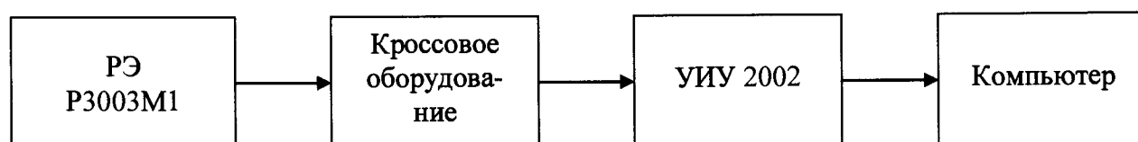
Рисунок 8 - Блок-схема поверки ИК напряжения постоянного тока, соответствующего значениям температуры
