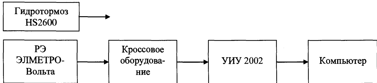
Рисунок 11 - Блок-схема поэлементной поверки ИК крутящего момента силы
