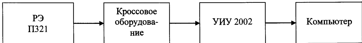
Рисунок 3 - Блок-схема поверки ИК силы постоянного тока, соответствующей значениям давления, в диапазоне от 4 до 20 мА
