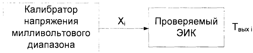
Рисунок 9.4 – Электрическая схема поверки ИК ПТК сигналов термопар
