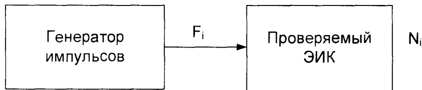
Рисунок 9.6 – Электрическая схема поверки каналов ПТК измерения частоты
