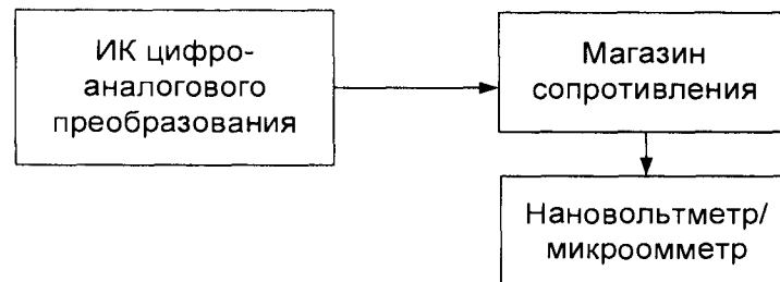
Рисунок 9.5 – Схема соединений при проверке основной погрешности канала ПТК цифро-аналогового преобразования
