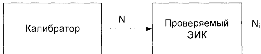
Рисунок 9.7 – Схема соединений при проверке основной погрешности ИК количества импульсов
