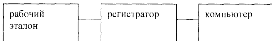
Рисунок 1 - Структурная схема подключения регистратора к внешним устройствам
