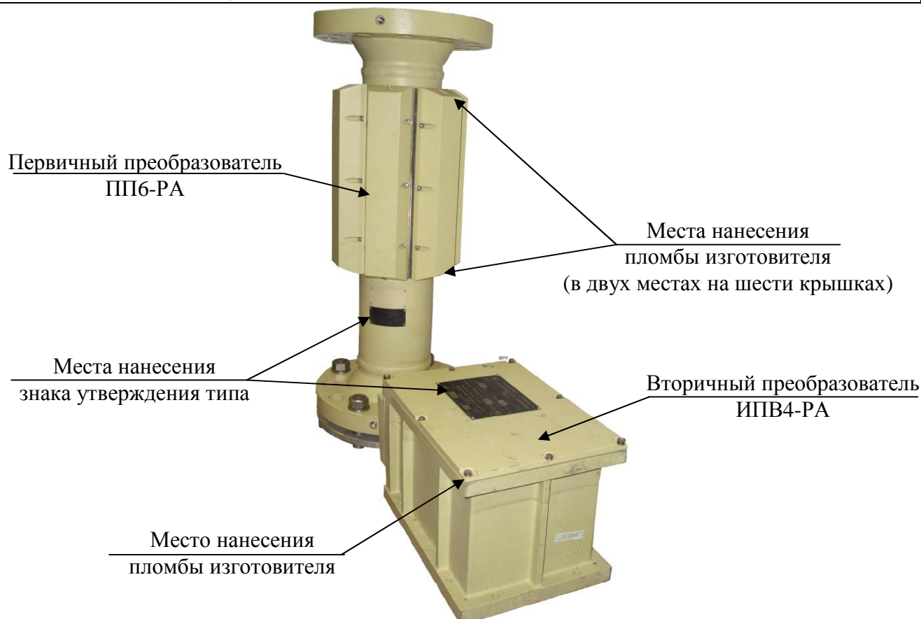
Рисунок 1 - Внешний вид расходомера
