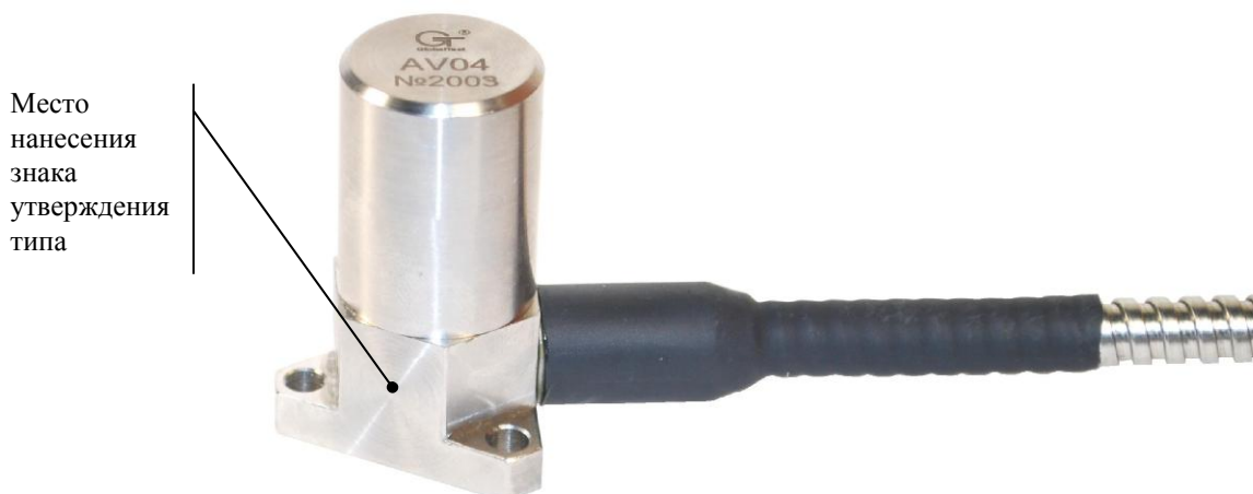
Рисунок 1 - Внешний вид датчика AV04
