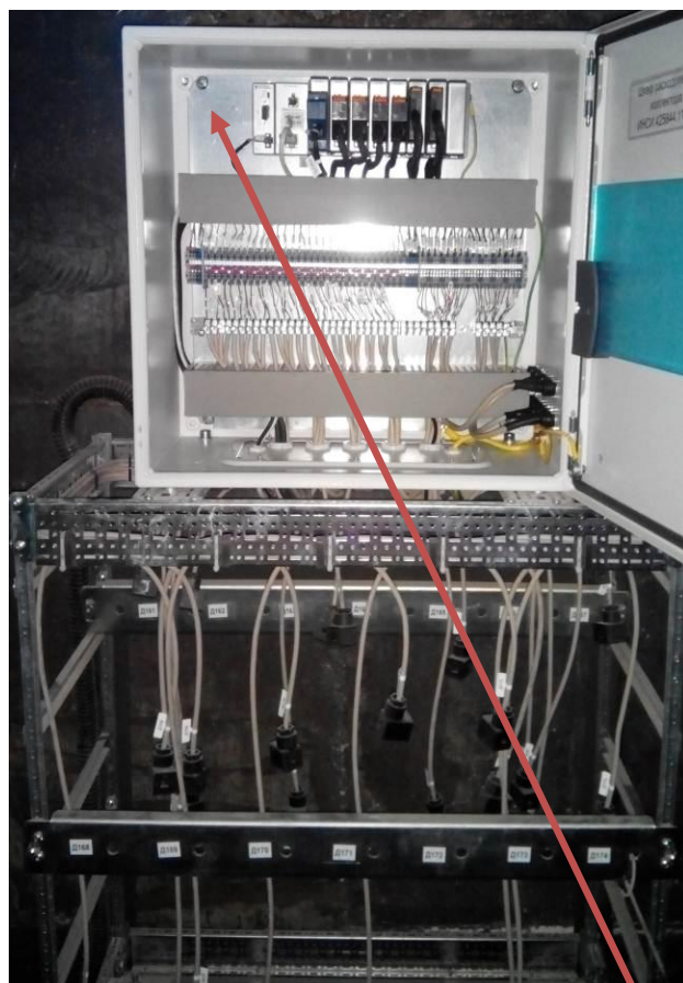
Рисунок 11 - Шкаф расходомерного коллектора 1
