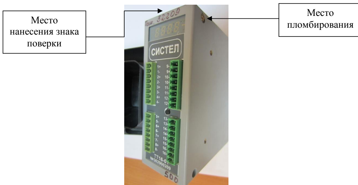
Рисунок 1 - Внешний вид, места нанесения знака поверки и пломбирования амперметров
