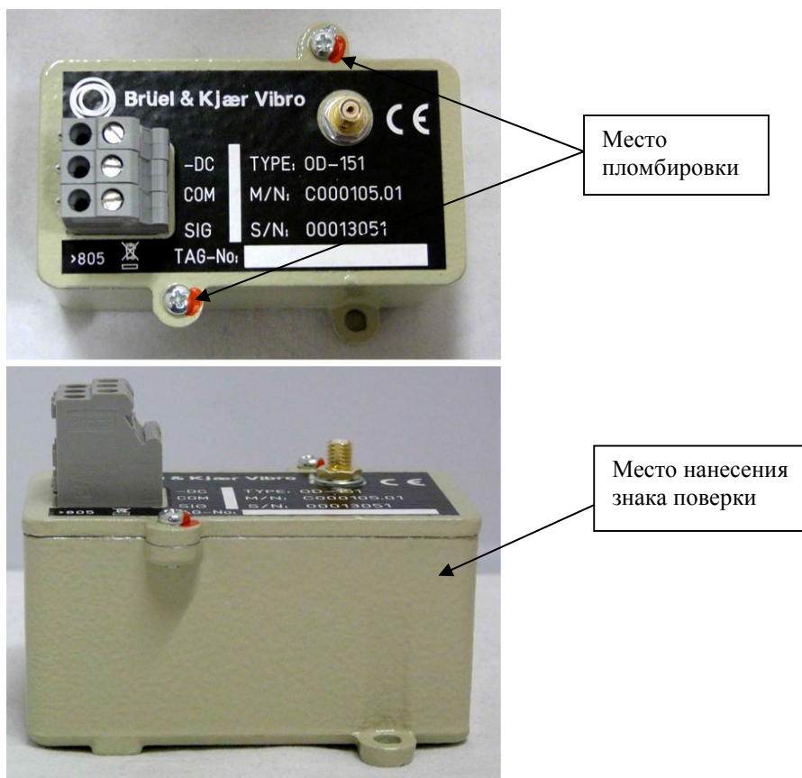
Рисунок 6 - Схема пломбировки осцилляторов модификаций OD-151, обозначение места нанесения знака поверки
