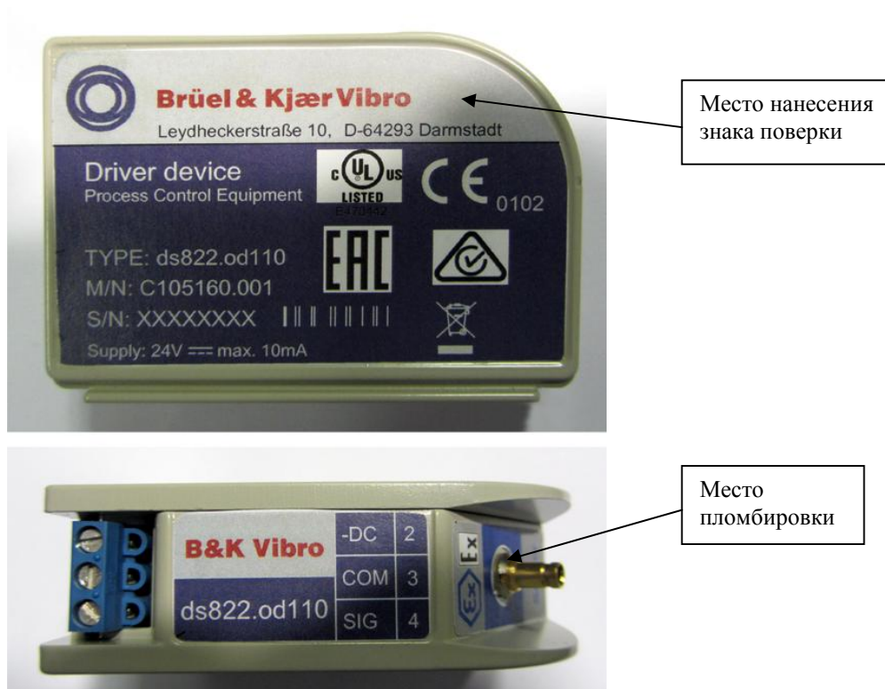
Рисунок 8 - Схема пломбировки осцилляторов модификаций ds82x.od110 и ds82x.od130, обозначение места нанесения знака поверки
