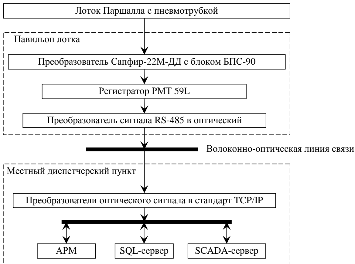
Рисунок 1 - Структура одного измерительного канала системы учета сточных вод Курьяновских очистных сооружений
