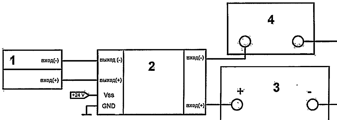
Рисунок А.3 – Схема соединения приборов при поверке входных аналоговых измерительных каналов типа 1 в составе с промежуточными измерительными преобразователями с гальванической развязкой (барьерами искробезопасности)
