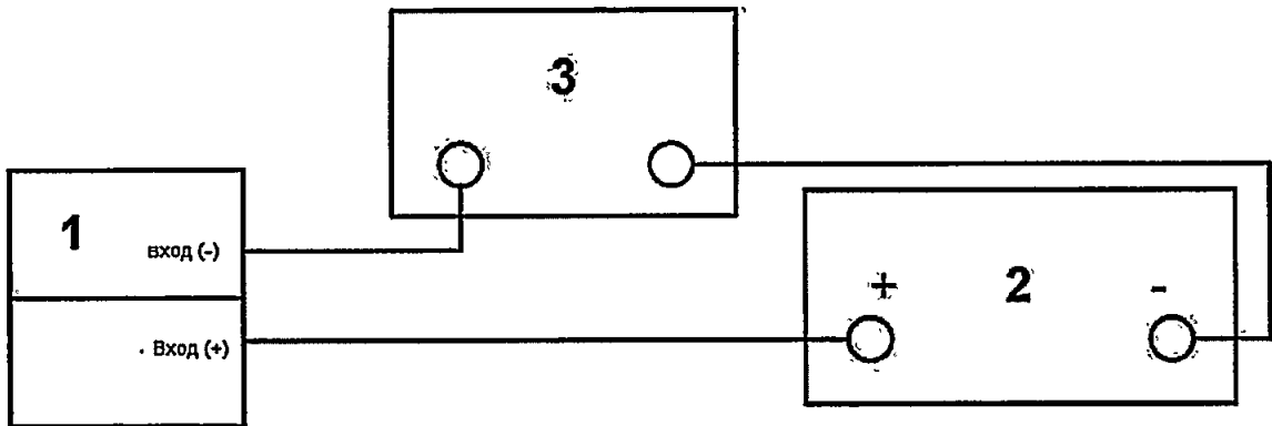
1 – модуль аналогового ввода; 2 –калибратор универсальный; 3 – магазин сопротивлений; Рисунок А.1 – Схема соединения приборов при поверке входных аналоговых измерительных каналов типа 2.
