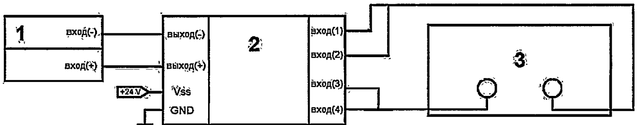
1 – модуль аналогового ввода; 2 – барьер искробезопасности; 3 – калибратор универсальный/магазин сопротивлений;
