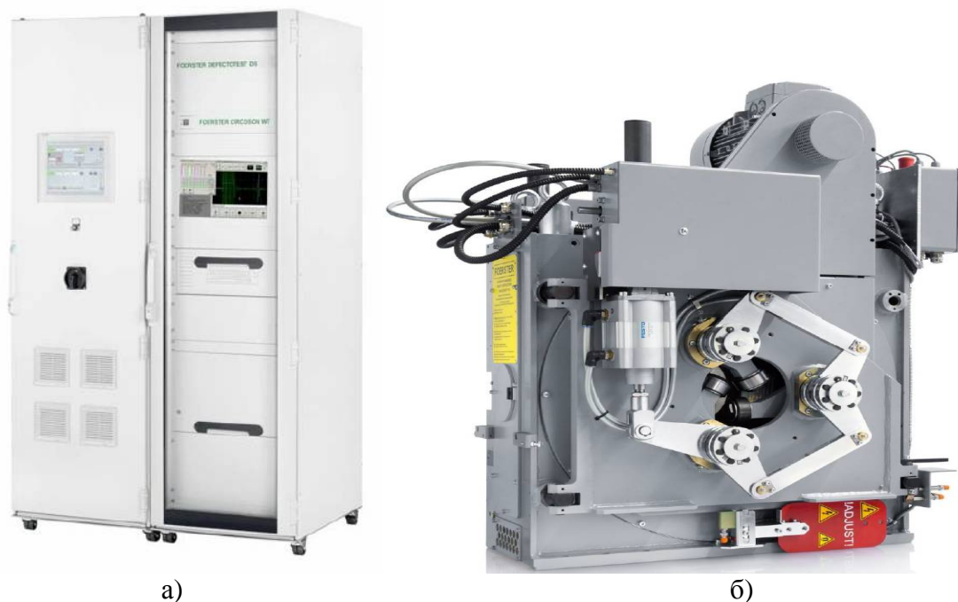
Рисунок 1 - Общий вид системы а) силовой шкаф и электронный шкаф; б) система датчиков Ro 180
