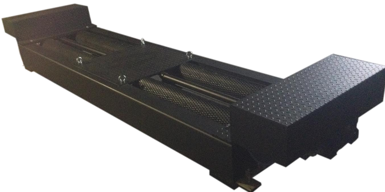
Рисунок 2 – Общий вид стенов тормозных РЕМСТО-ТС-13-1С-1-7.5Ч
