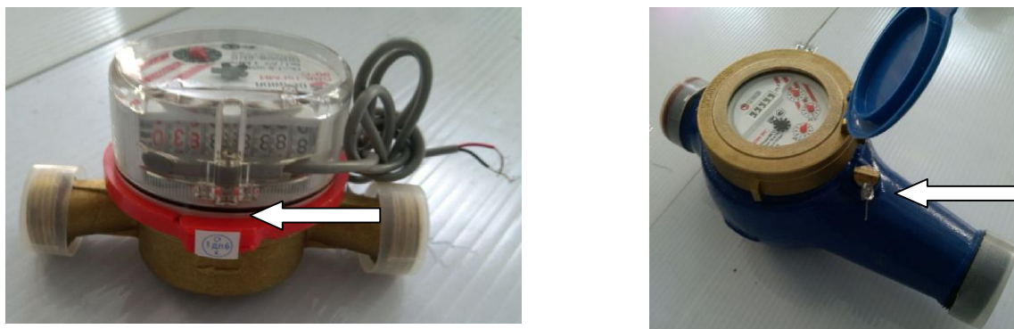
Рисунок 2 - Схема пломбировки от несанкционированного доступа, обозначение места нанесения знака поверки счетчиков воды крыльчатых СВК, СВКМ
