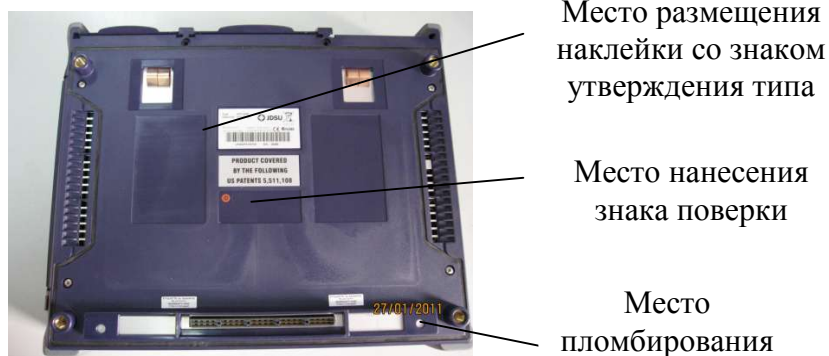
Рисунок 3 - Схема пломбировки от несанкционированного доступа, место размещения наклейки со знаком утверждения типа и знака поверки базового блока модификации MTS-8000E
