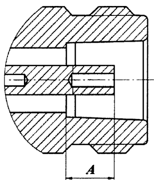
N, розетка
