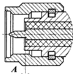
SMA, вилка
