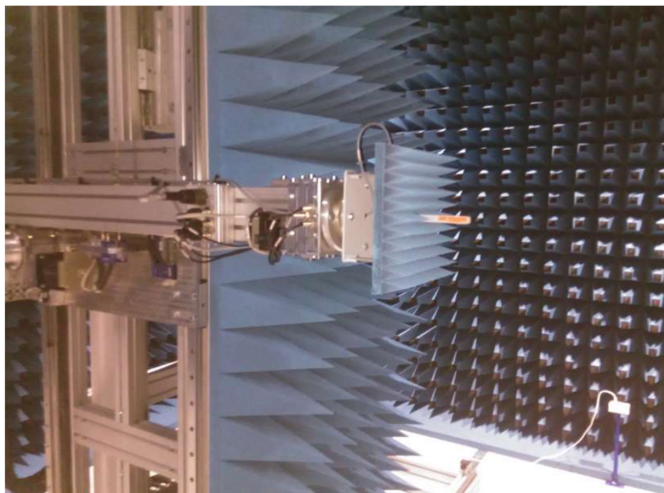
Рисунок 3 - Внешний вид сканера (ось Z) с установленной антенной-зондом
