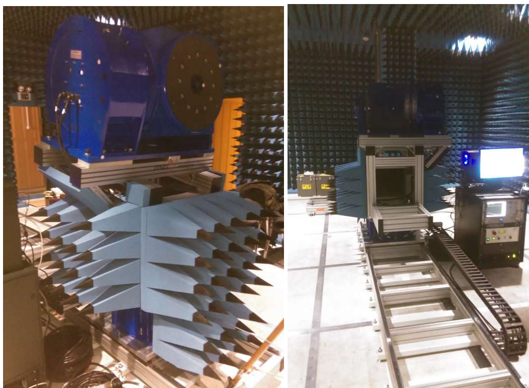
Рисунок 2 - Внешний вид позиционера
