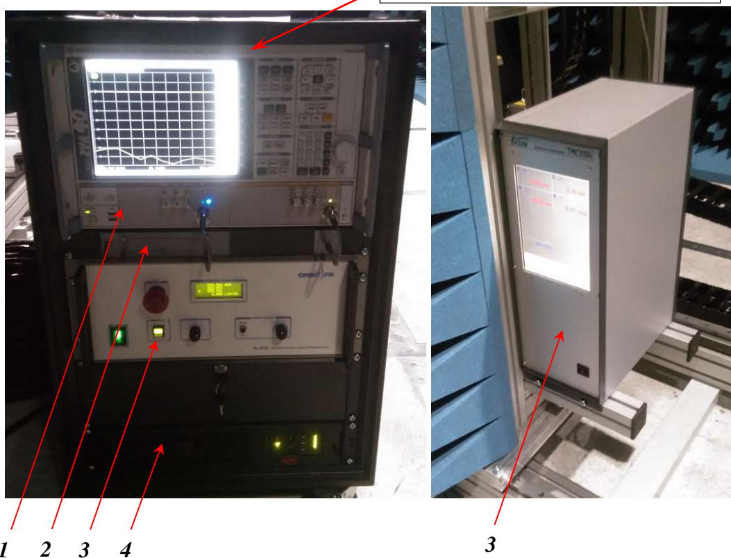
Рисунок 4 - Внешний вид векторного анализатора цепей (1), комплекта малошумящего усилителя (2), контроллеров движения (3), источника бесперебойного питания (4)
