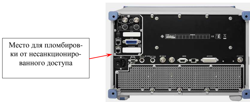
Рисунок 9 - Задняя панель векторного анализатора цепей
