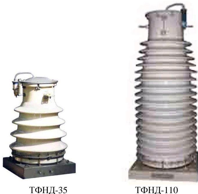
Рисунок 1 - Фотографии общего вида трансформаторов тока ТФНД
