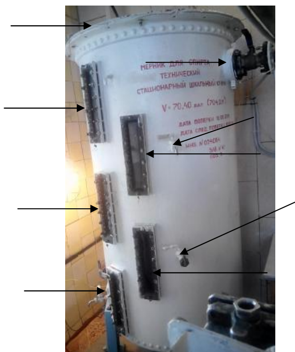
Рисунок 1 - Общий вид и места пломбирования мерника
