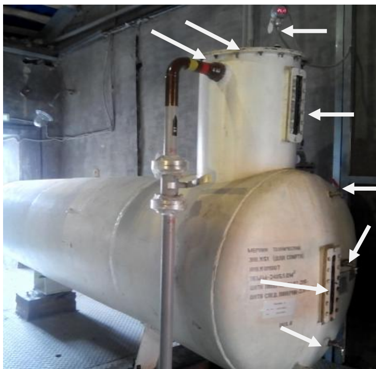
Рисунок 1 - Общий вид и места пломбирования мерника
