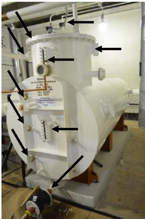
Рисунок 1 - Общий вид и места пломбирования мерника
