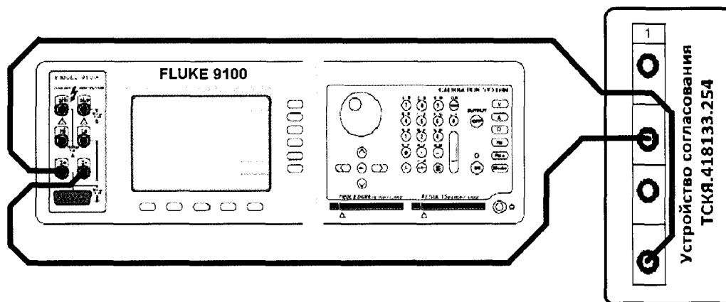
Рисунок 26 – Схема определения абсолютной погрешности измерения силы тока источником питания MS DPS на пределах 0,3; 4; 8А
