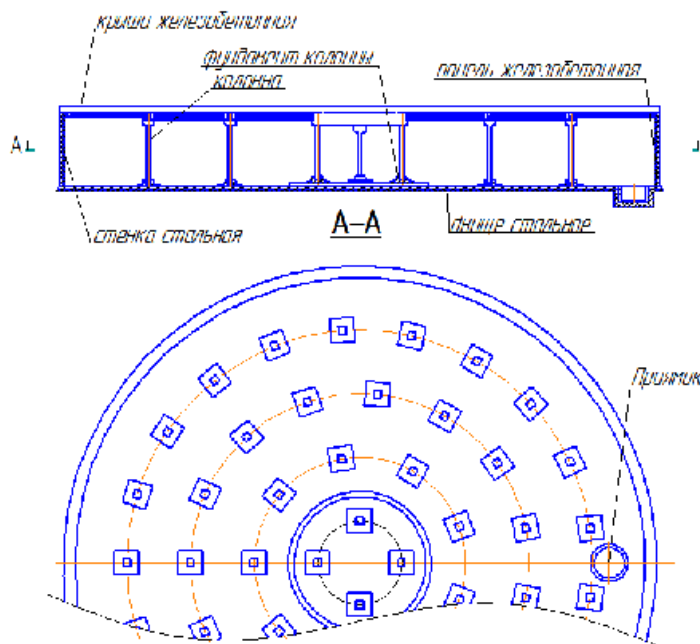
Рисунок 1 - Эскиз резервуара
