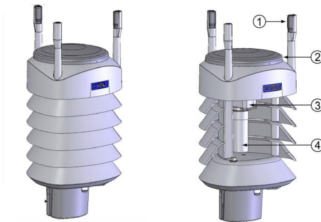
Рисунок 1 - Общий вид метеостанций WXT530
