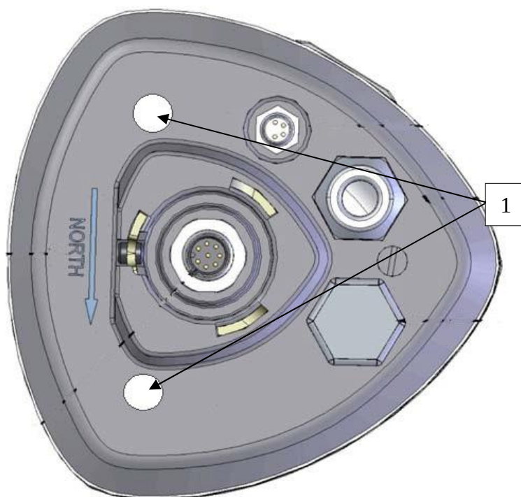
Рисунок 3 - Схема пломбирования метеостанций WXT530
