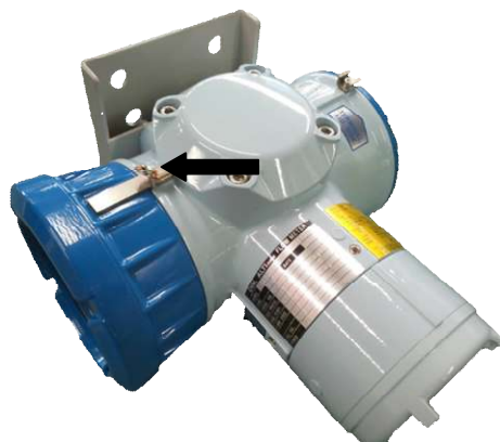
Рисунок 2 - Общий вид и место пломбирования вторичного преобразователя расхода счетчиков-расходомеров массовых кориолисовых OVAL модификаций ALTI mass Type U, ALTI mass Type S и ALTI mass Type B
